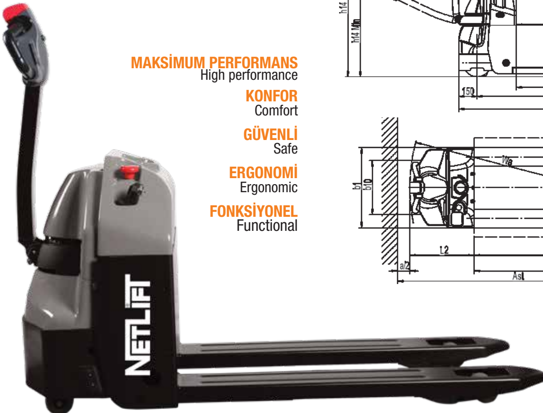
DAHİLİ ŞARJ CİHAZI INTERNAL CHARGER
